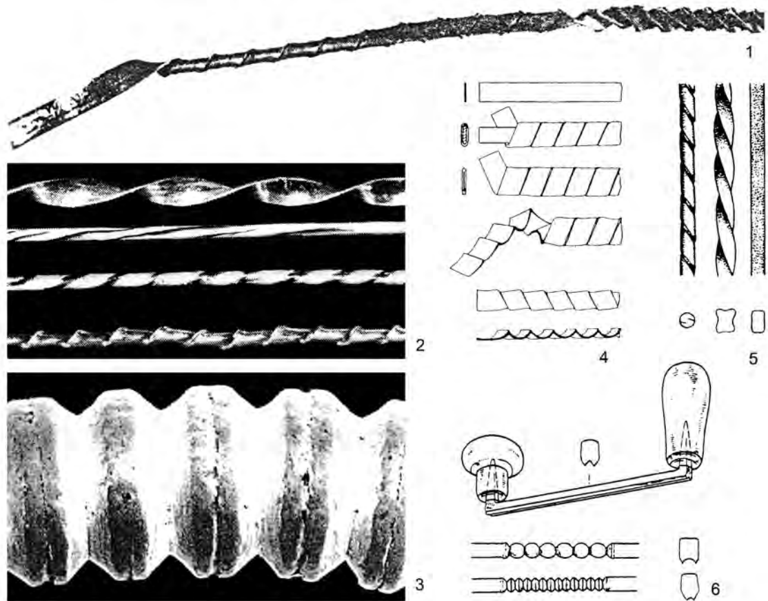
Abb. 13 — Drahtherstellung: 1, 4, gerippter Blechstreifen; 2, 5, Wendeldraht als Ausgangsform für einen Spiralspuldraht; 3, Perldraht mit äquatorschnitt; 6, Perldraht.
