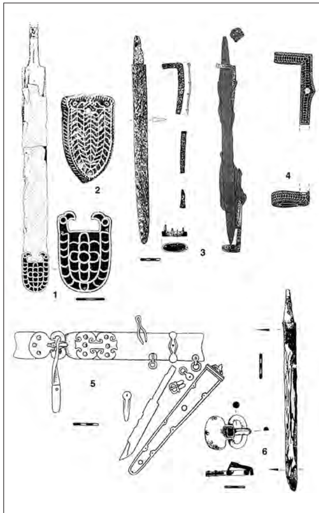
Fig. 6 - Les scramasaxes et les épées courtes du Ve s. 1.- Zaragiž. 2.- Boulerolle de l'épée de Childéric. 3.- Eschborn. 4.- Fourreau du scramasaxe de Childéric. 5.- Sapka-Justinianov Holm. 6.- Kosarevo (d'après Kazanski, Mastykova, Périn 2002).
